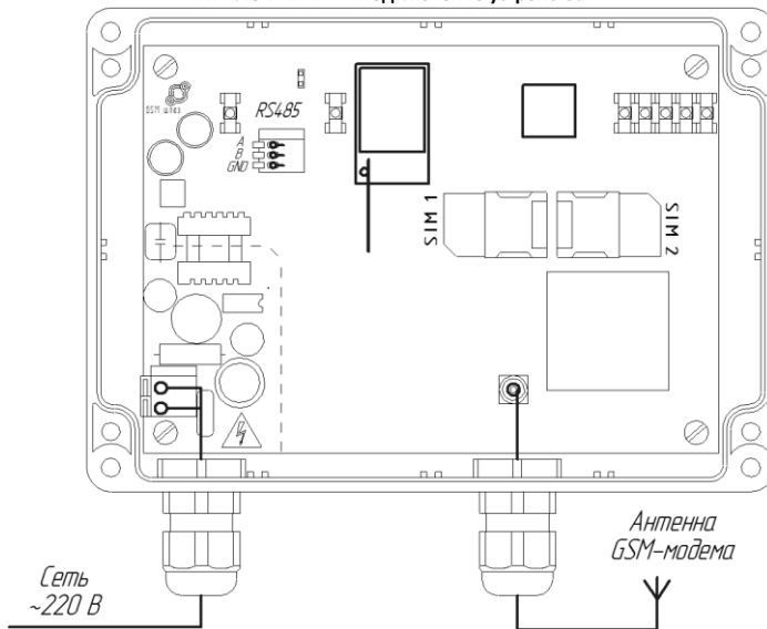
ПРИЛОЖЕНИЕ В - Подключение устройства
